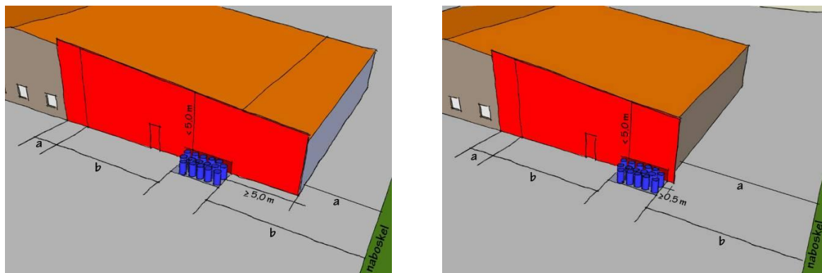
Figur 37: Eksempel på bortfald af den indbyrdes afstand, ved oplag mod bygning, ved etablering af brandsektionsadskillelse inden for den krævede afstand. "Den krævede afstand" svarer til den indbyrdes afstand fundet vha. "sumreglen". I figuren til venstre skal der ikke etableres sikring mod brandsmitte i gavlen, da afstanden overstiger 5 m. I figuren til højre er der vist sikring mod brandsmitte i gavlen, idet brandsektionsadskillelsen er videreført til en afstand af 0,5 m fra bygningens ydervæg. Der er udført en brandkam, idet afstanden fra oplaget til taget er mindre end 5 m.
