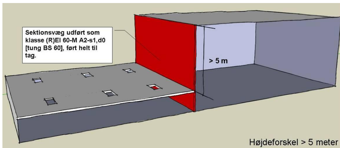
Figur 28: Sikring mod høj-lav brandsmitte, hvor den højere bygnings tag er større end 5 m over den lavere bygnings tag. Ingen krav om brandkam eller brandkammerstatning.
