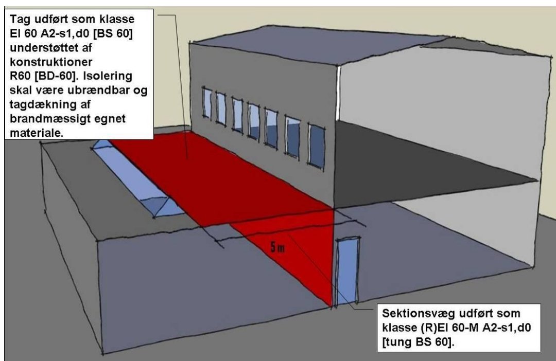
Figur 29: Sikring mod høj-lav brandsmitte, hvor sikringen er udført på den lavere brandsektions tag. Der henvises til vejledningens afsnit om brandkammerstatning for udførelse af tagdækning i brandmæssigt egnet materiale.
