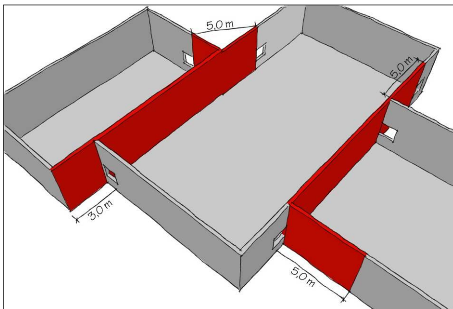
Figur 25: Eksempler på sikring mod vinkelsmitte i ydervægge.
