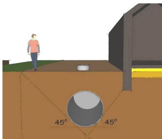
Figur 16: Trykzonen i forhold til bygninger, naboskel og vej kan fastlægges ud fra en 45^\circ vinkel.
