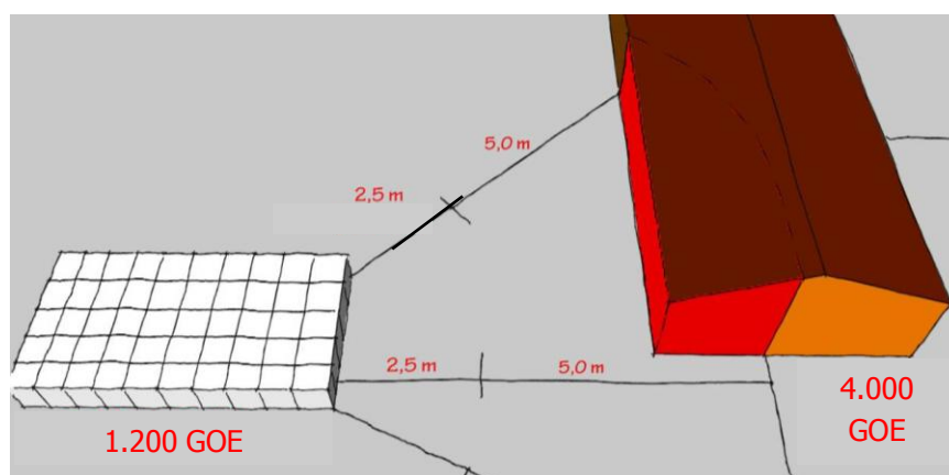
Figur 38: Nedsættelse af den indbyrdes afstand ved oplag mod bygning ved etablering af brandsektionsadskillelse i facaden inden for den krævede afstand (i dette eksempel 7,5 m). Sikring af tag og særlige foranstaltninger mod brandsmitte på gavlvæggen skal kun ske, når den indbyrdes afstand er mindre end 5 m.
