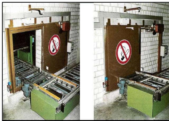
Figur 31: Billede af en transportåbning.
