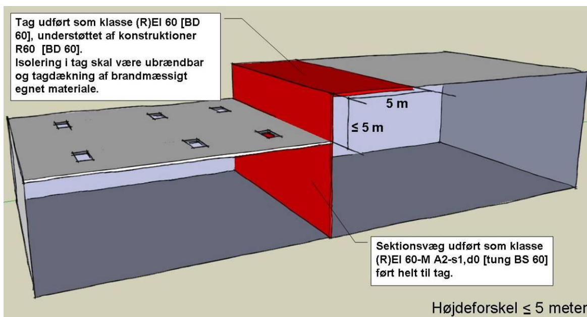
Figur 27: Sikring mod høj-lav brandsmitte, hvor den højere bygnings tag er mindre end eller lig med 5 m over den lavere bygnings tag. Løsning med brandkamserstatning. Der henvises til vejledningens afsnit om brandkamserstatning for udførelse af tagdækning i brandmæssigt egnet materiale.
