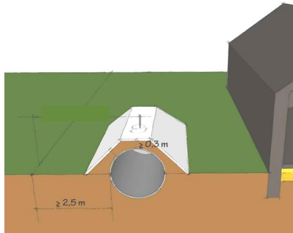
Figur 14: Tank, der er forsynet med en belægning eller lignende, som sikrer, at jordlaget forbliver intakt og dermed bevarer jordlagstykkelsen.
