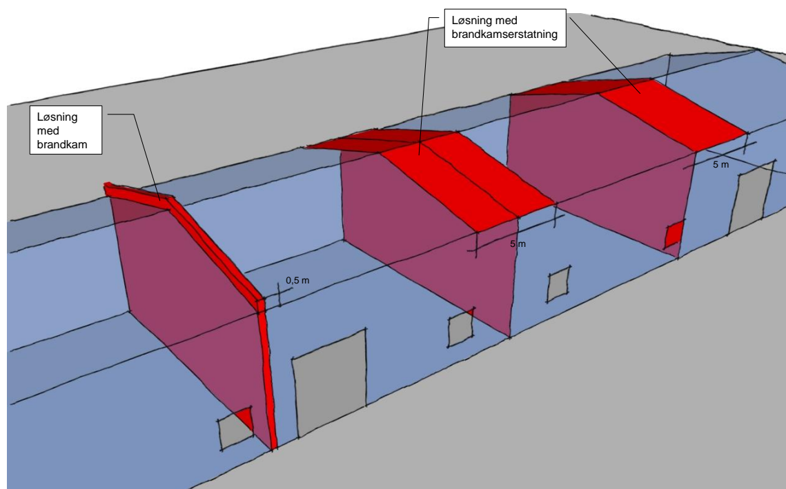
Figur 22: Illustration af løsning med hhv. brandkam, dobbeltsidet og enkelsidet brandkamserstatning.
