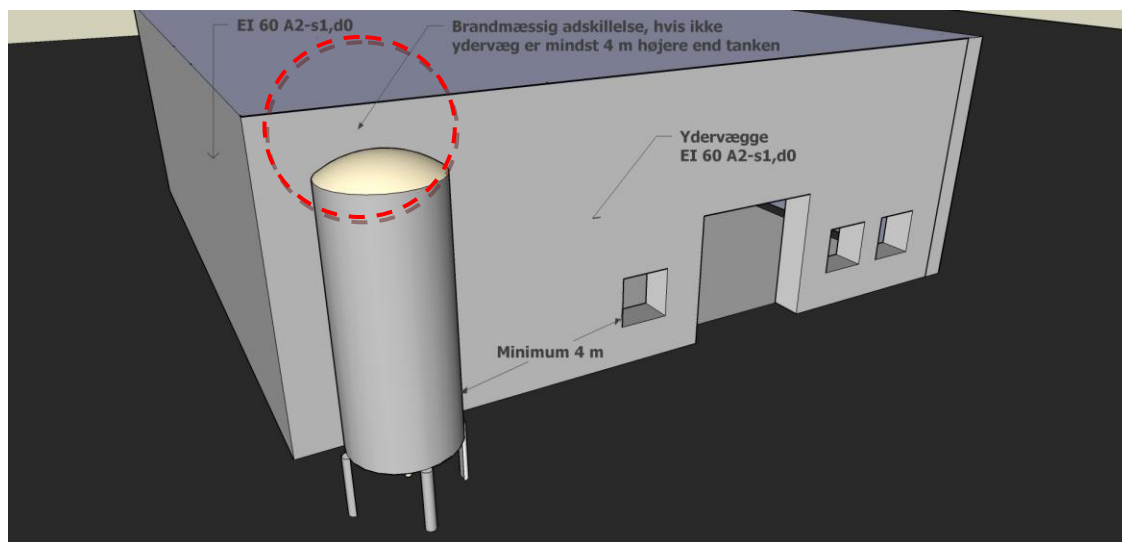
Figur 17: Illustration af afstandsforhold for kryotanke med inaktive eller brandnærende gasser i forhold til en bygning, der ikke er omfattet af beredskabslovgivningen.
