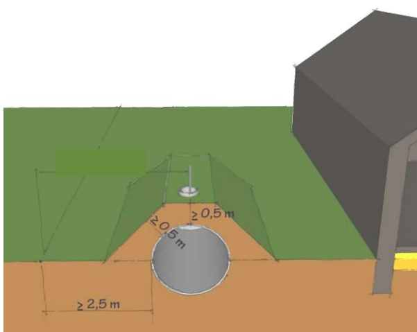
Figur 13: Tank, der er jorddækket med mindst 0,5 m jord.
