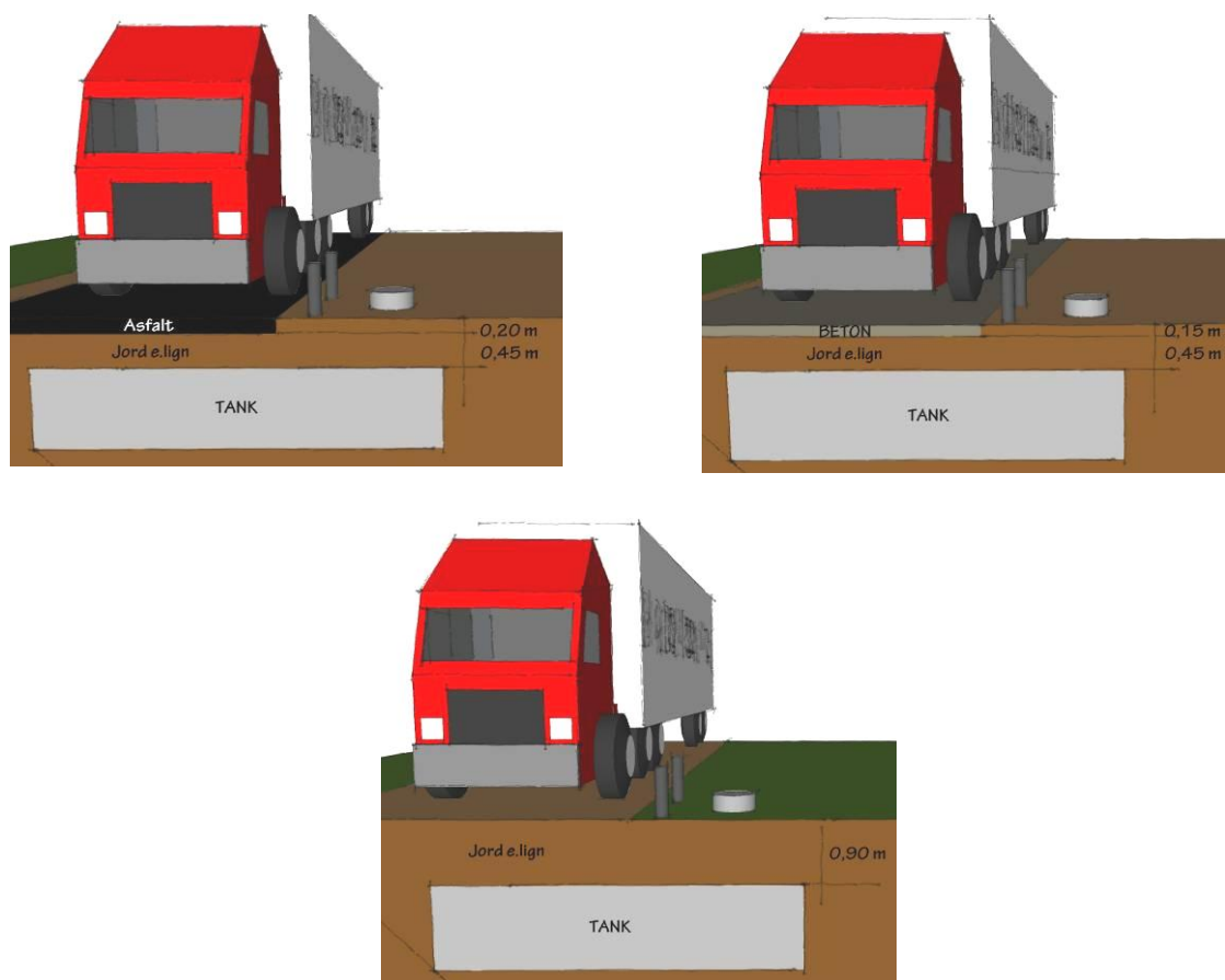
Figur 15: Illustration af forskellige belægningsmuligheder, herunder tykkelse til beskyttelse af tanken mod trafiklast.
